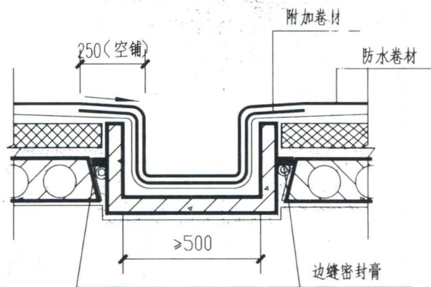
4 预制屋面中天沟
