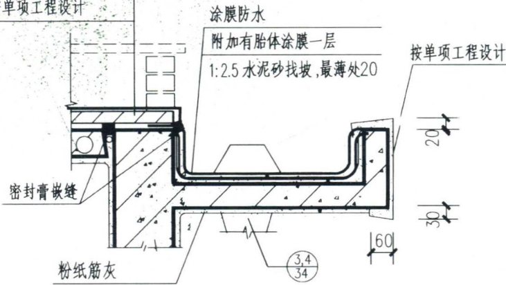
③ 现浇天沟檐口
