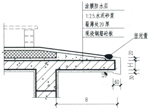
① 平檐口
