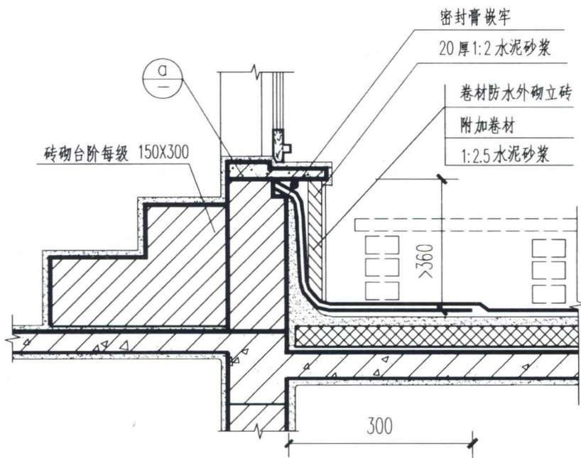
1 无变形缝出入口(一)
