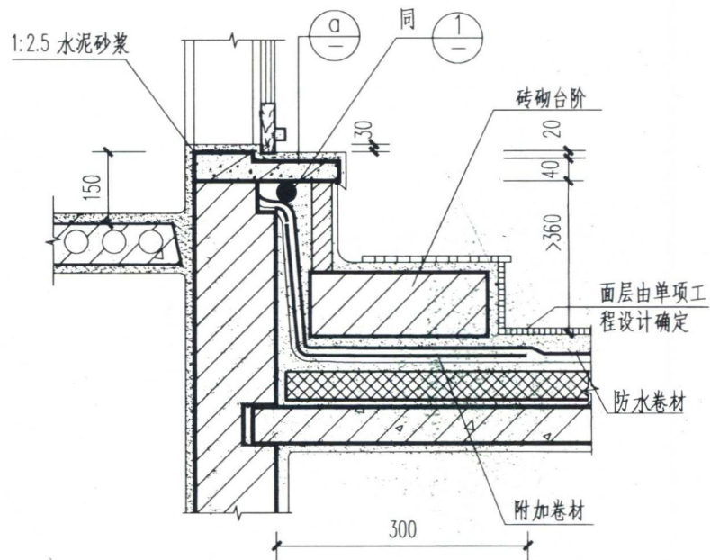
2 无变形缝出入口(二)
