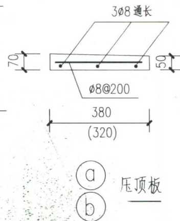
3 帶斜板天沟
