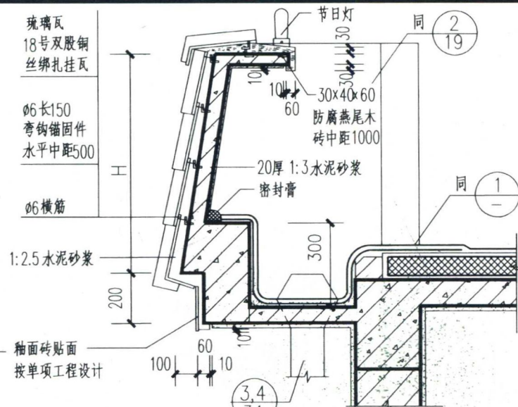
③ 带斜板天沟 (一)
