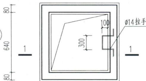
③ 钢筋砼检修孔
