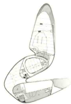
三层平面图 second floor plan
