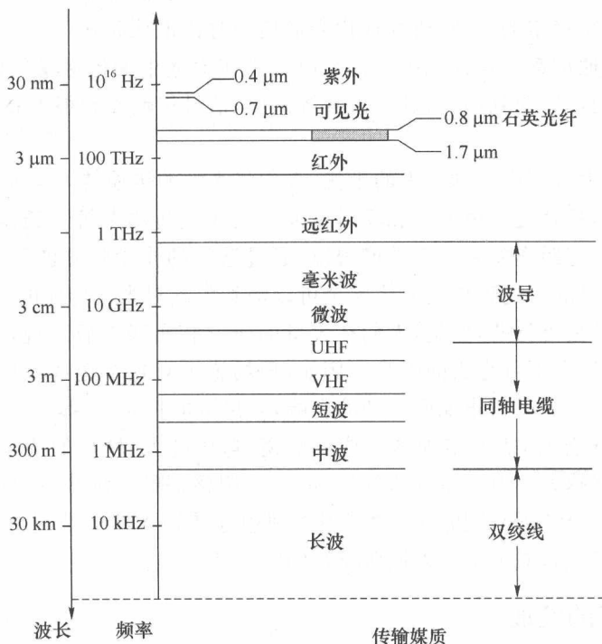
图 1.1.1 电磁波谱
