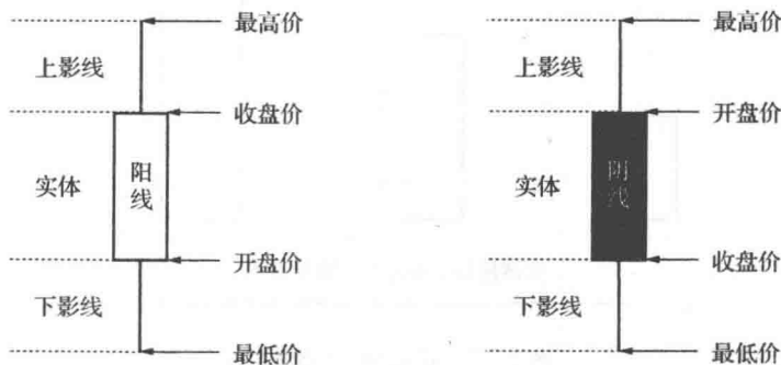
图 1—4 阳线和阴线
