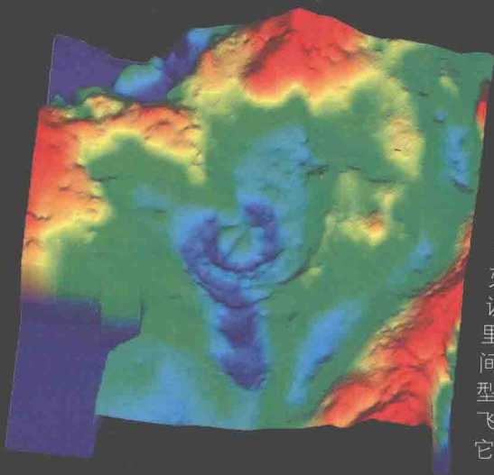
希克苏鲁伯陨石坑
