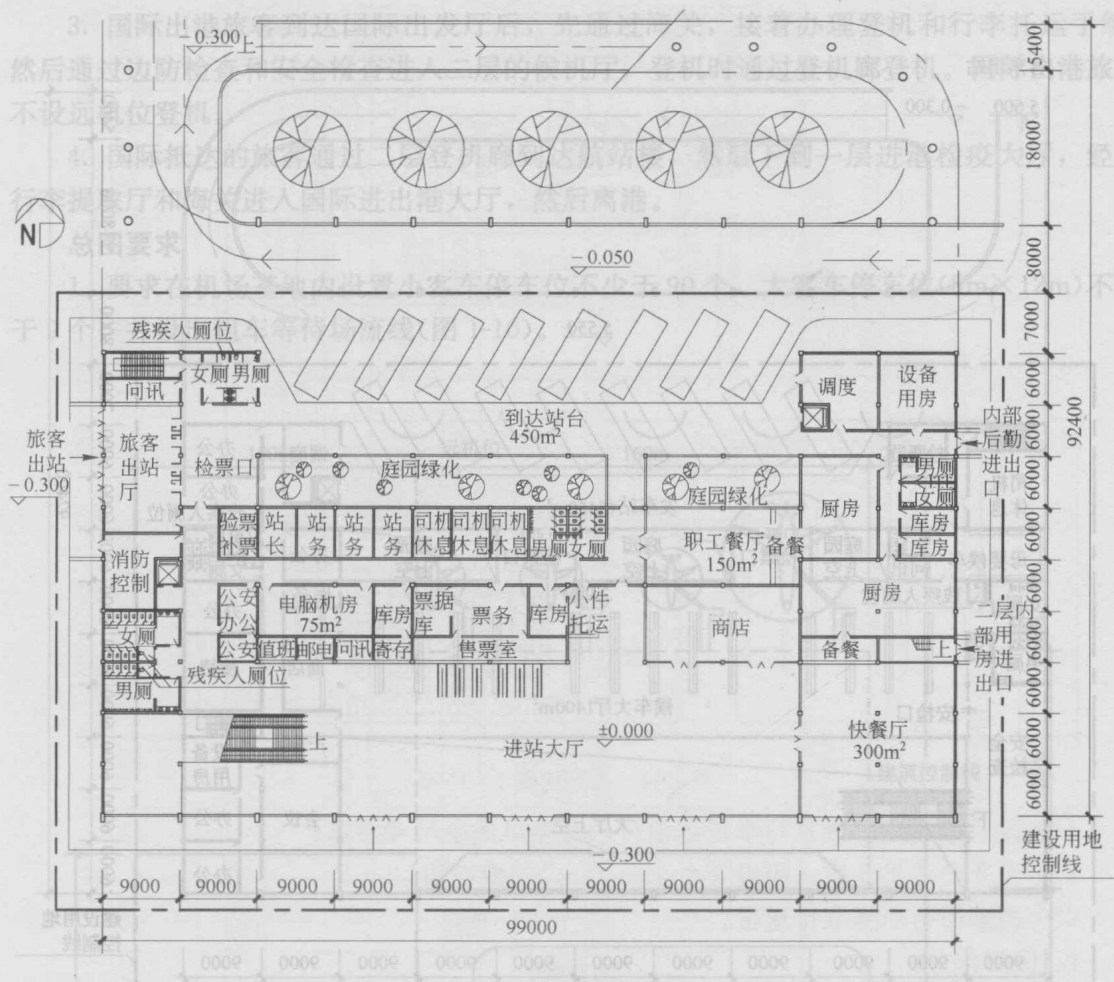
图 1-8 一层平面图 1:800
