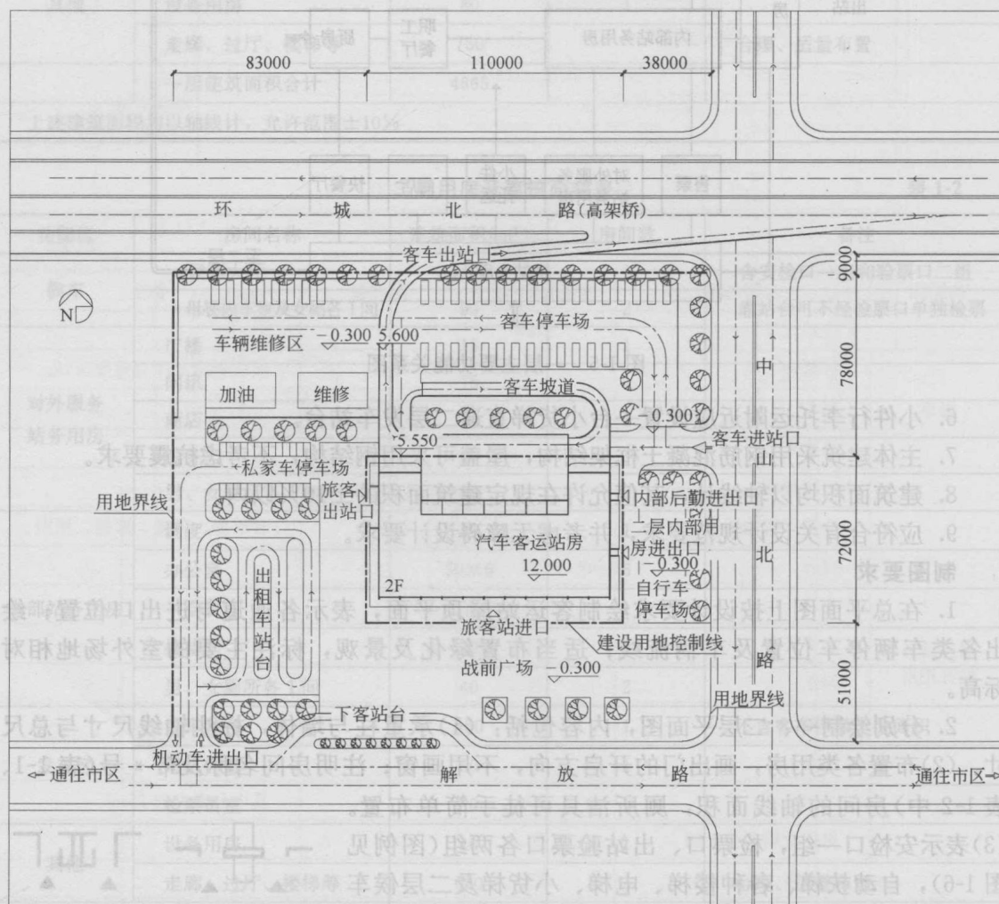
图 1-7 总平面 1:2500
