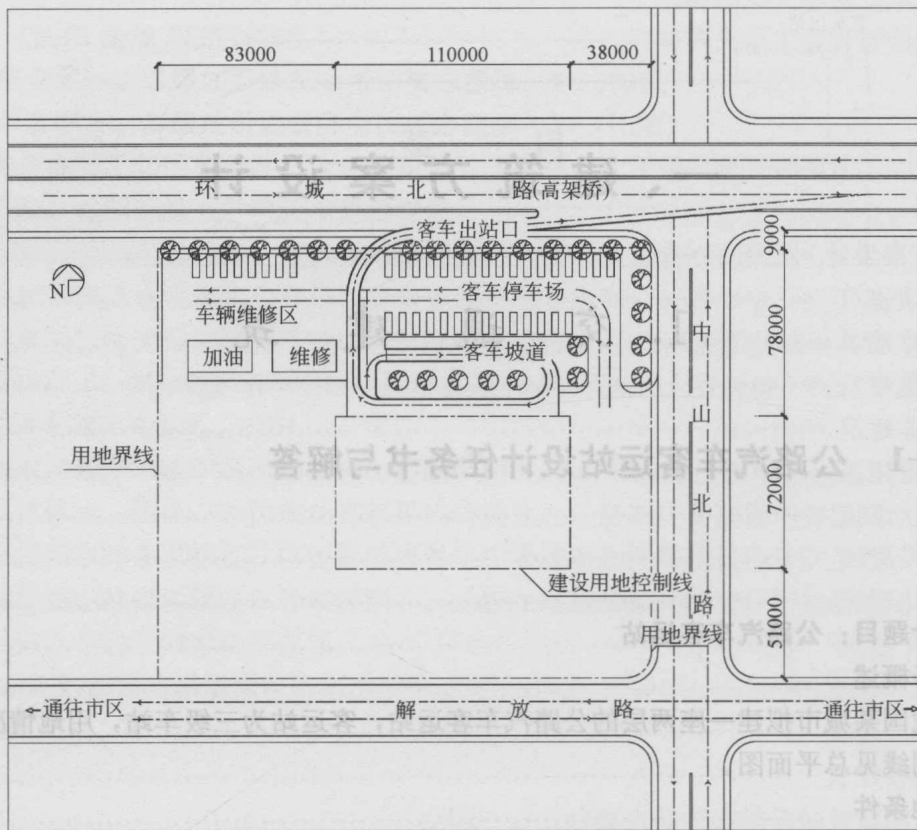
图 1-1 总平面图 1:2500
