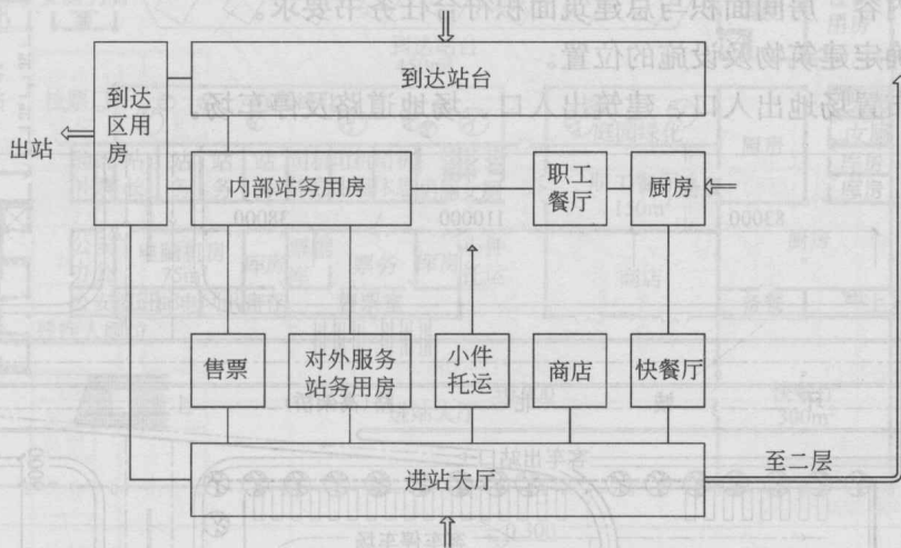
图 1-5 一层主要功能关系图
