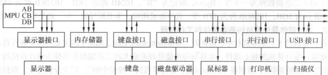
图 1.4 微型计算机的硬件系统结构示意图
