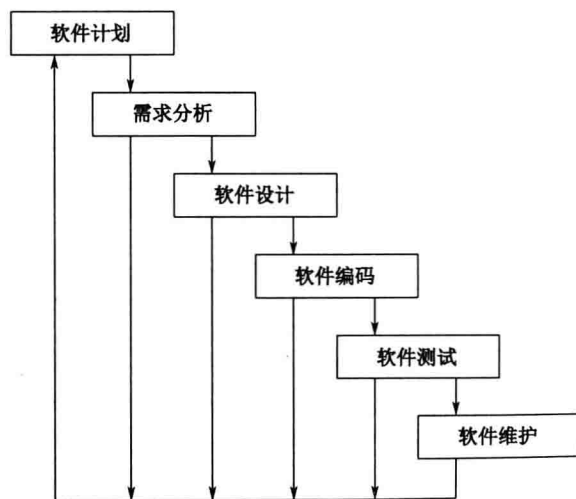
图 1-1 瀑布模型
