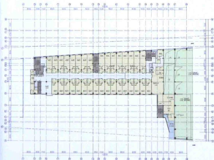
B区配套区四层平面图
