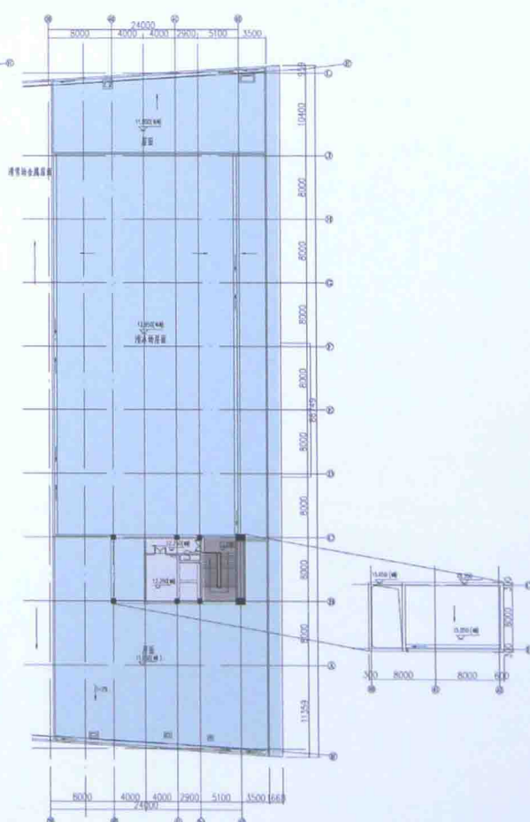
D区服务区屋面平面图
