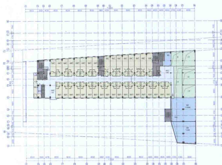
B区配套区三层平面图
