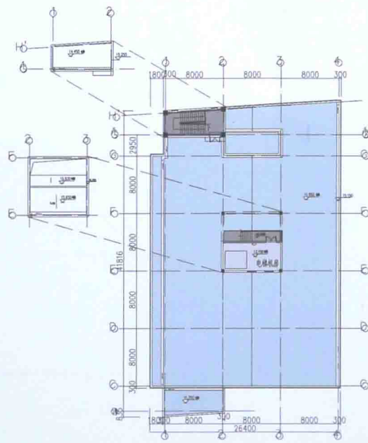
A 区体检中心屋面平面图
