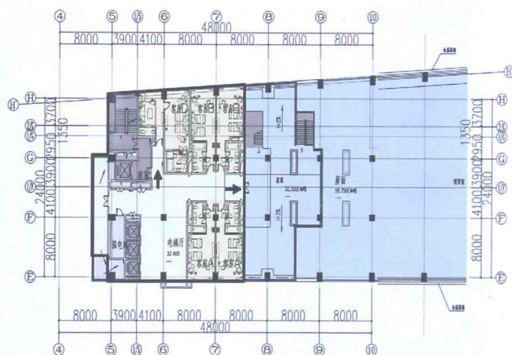
B 区配套区九层平面图
