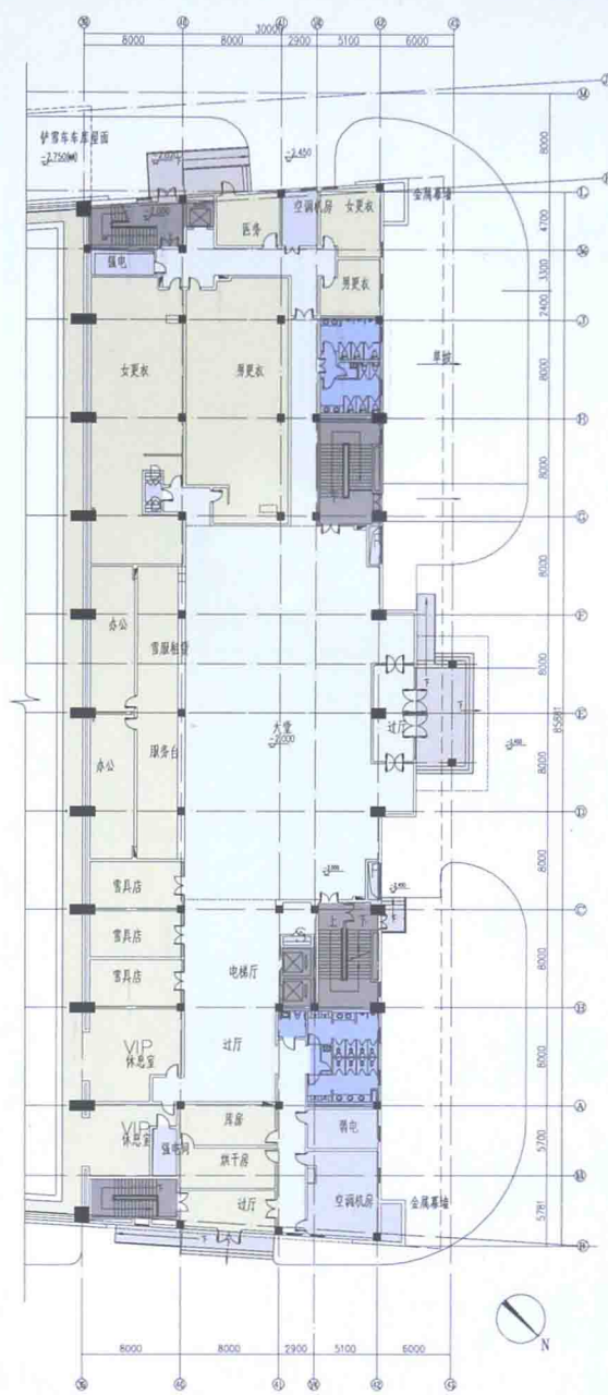
D 区服务区一层平面图
