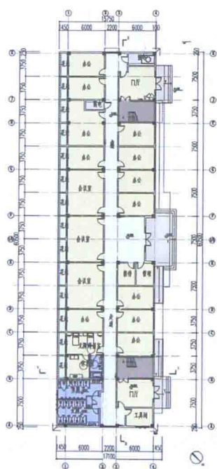
F区宿舍一层平面图
