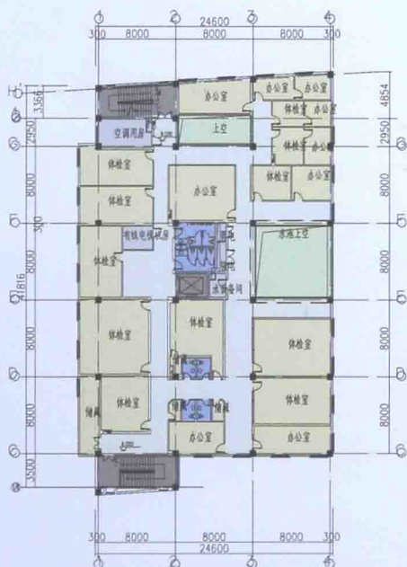
A 区体检中心三层平面图
