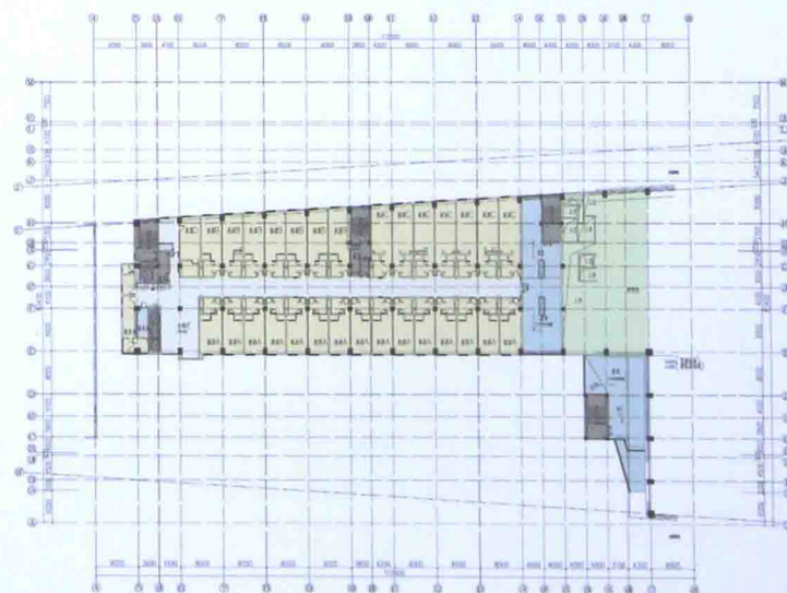
B区配套区五层平面图
