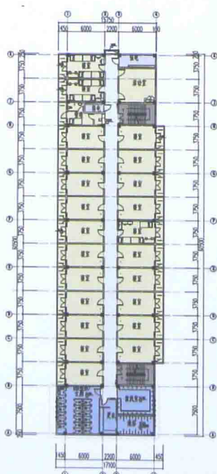
F区宿舍四层平面图
