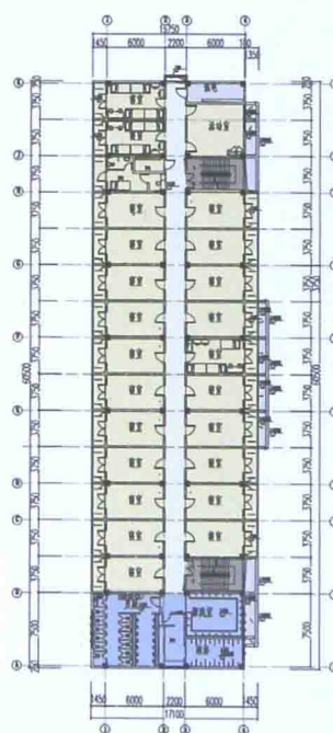
F区宿舍二层平面图
