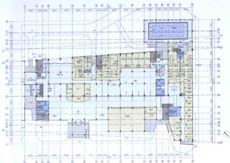
B区配套区一层平面图
