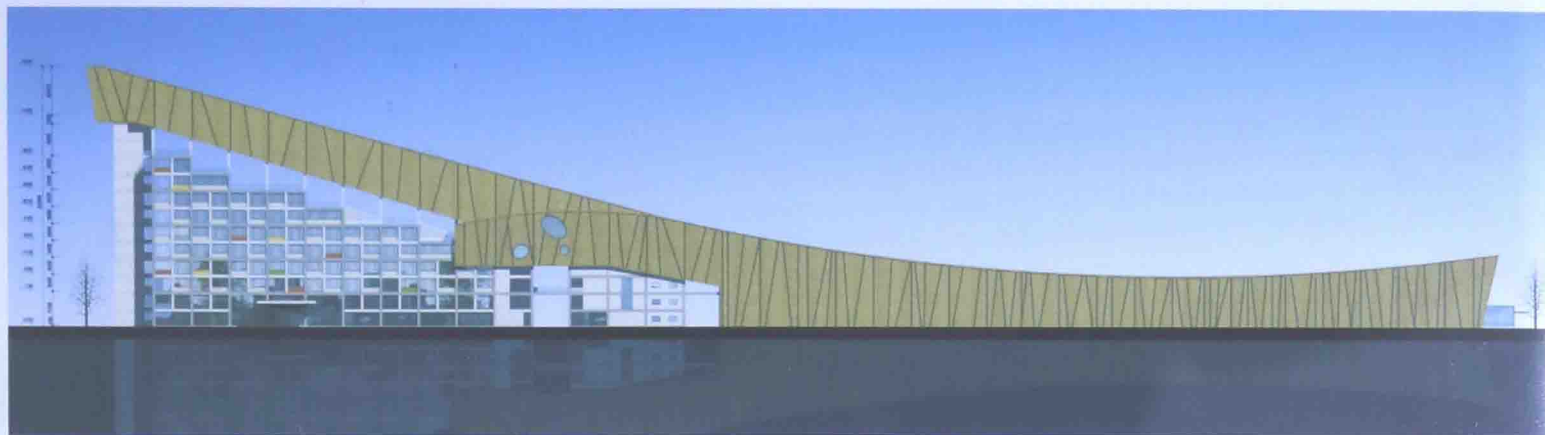
乔波冰雪世界立面图、剖面图
