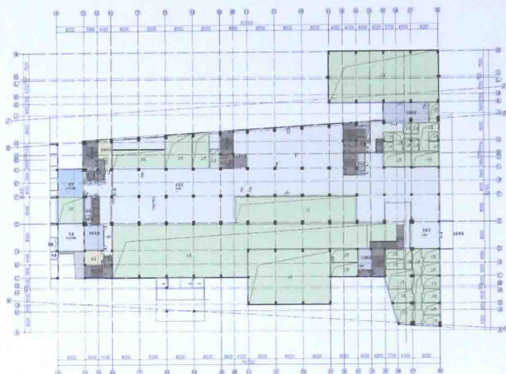
B区配套区夹层平面图
