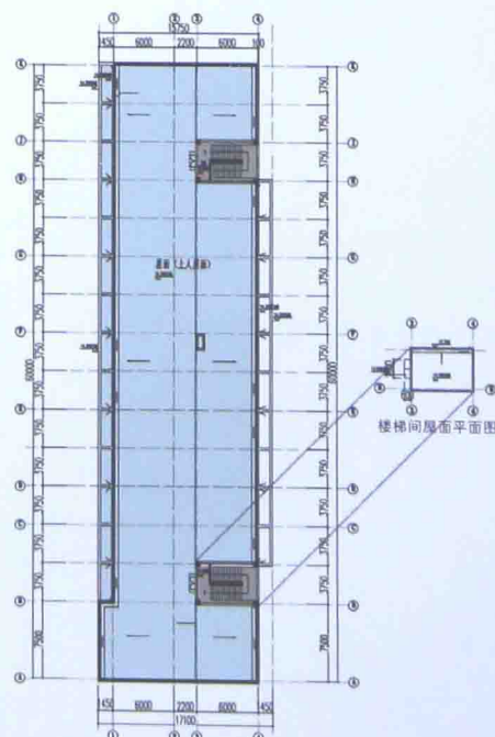
F区宿舍屋面平面图
