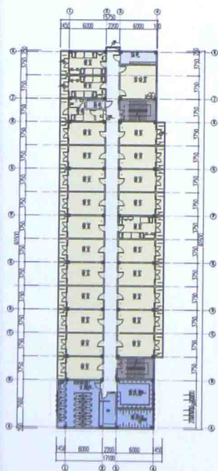
F区宿舍三层平面图
