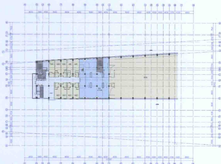
B 区配套区八层平面图
