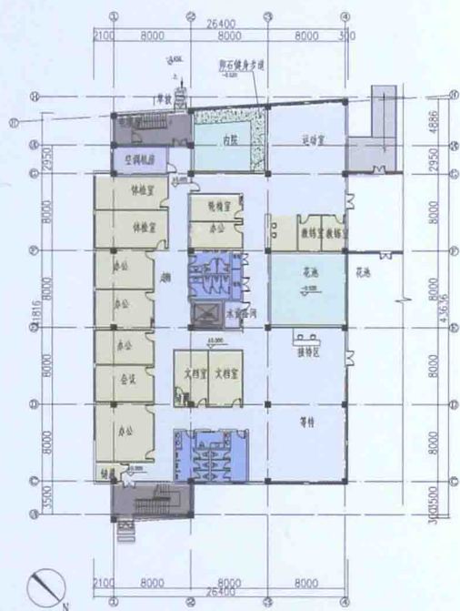
A 区体检中心一层平面图
