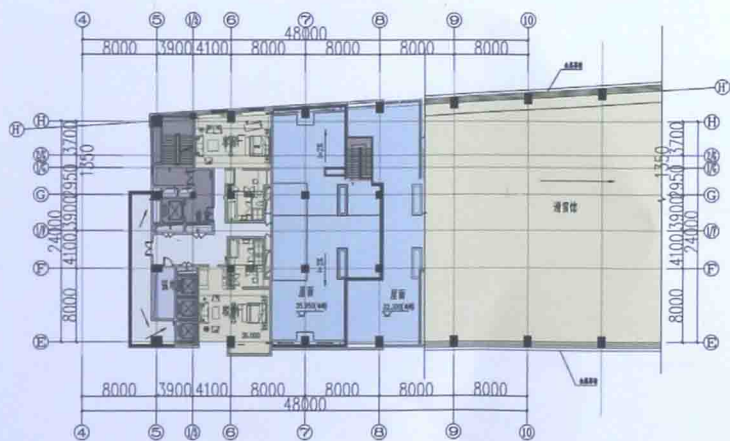
B 区配套区十层平面图
