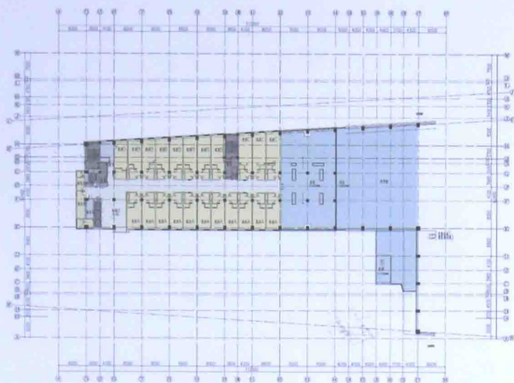
B 区配套区六层平面图
