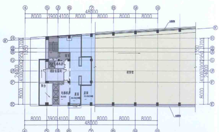
B 区配套区十一层平面图
