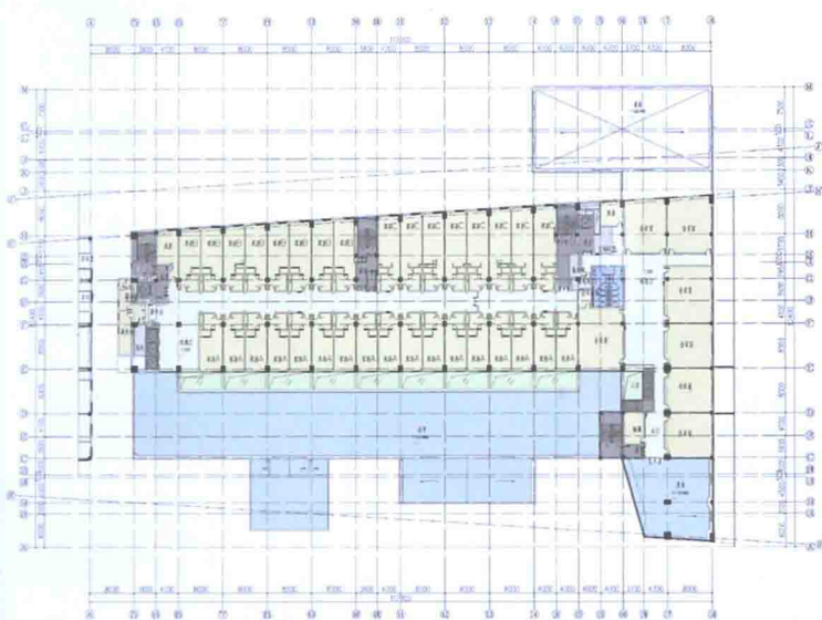
B区配套区二层平面图
