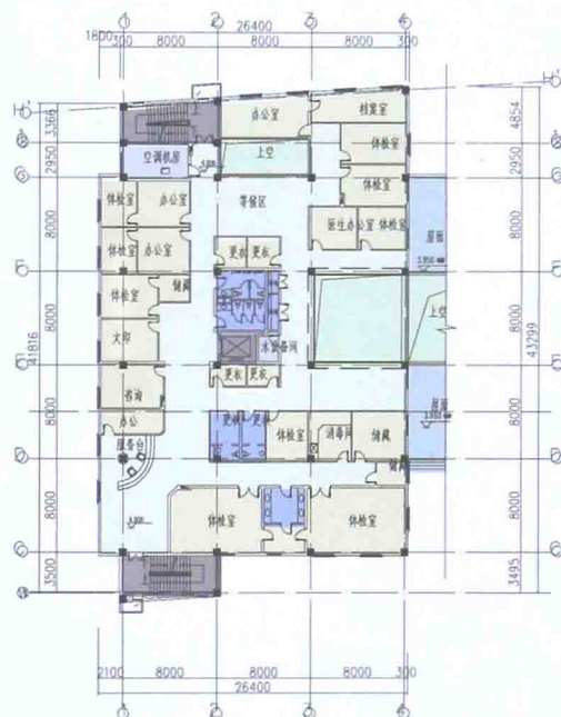
A 区体检中心二层平面图
