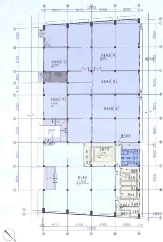
C区设备机房区一层平面图
