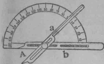
圖八 接觸測角器
