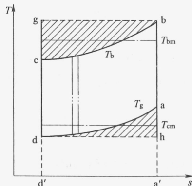
图 1-2 变温热源条件下可逆的逆向循环
