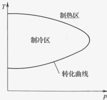
图 1-1 转化曲线
