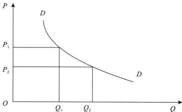
图 1-1 需求曲线
