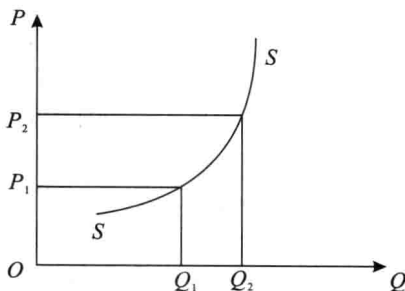
图 1-2 供给曲线
