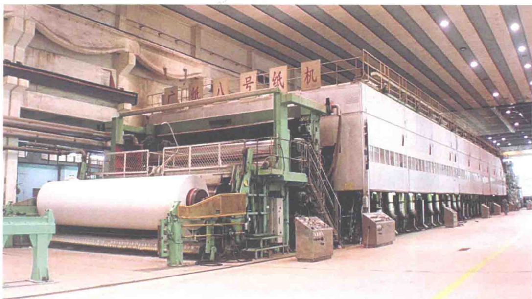
●广州造纸有限公司从瑞典引进的夹网新闻纸第八号纸机（抄宽8300毫米，运转速度达1000米/分钟），2000年投产，是全国新闻纸行业中规模最大的纸机
