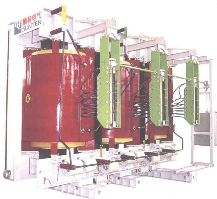
●1991年，顺德特种变压器厂生产的干式变压器
