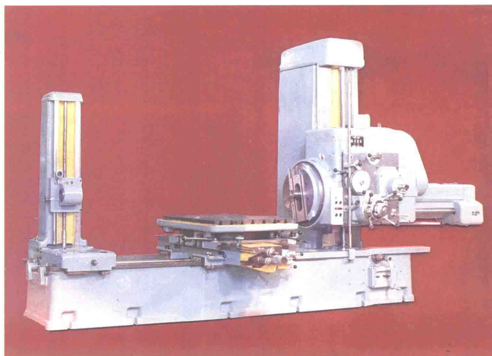
● 1979—1985年间，广州第三机床厂生产的T68型卧式镗床
