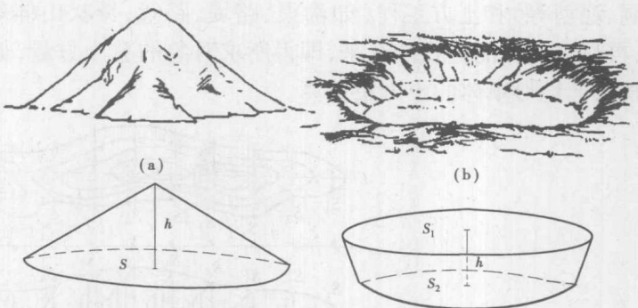
图 1.8 近似规则图形估算土方量
