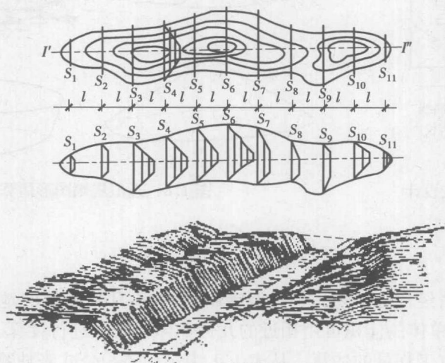
图 1.9 带状土山与沟渠、路堑垂直断面取法
