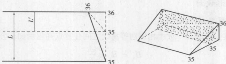
图 1.3 缩小等高线间距使地形坡度变陡
