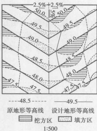
图 1.7 平整场地的等高线设计
