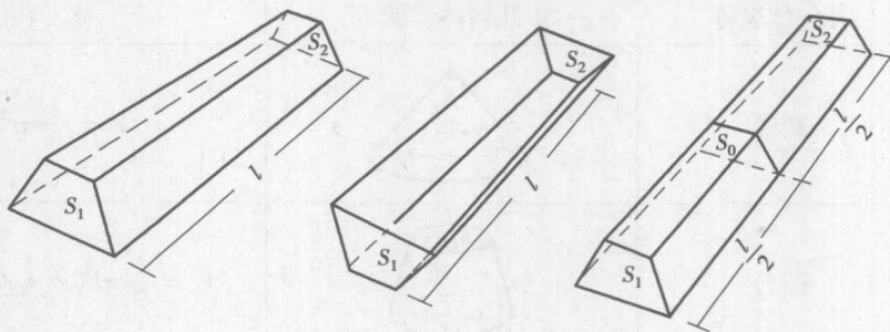
图 1.10 求中截面积
