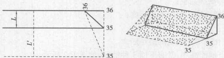
图 1.4 增大等高线间距使地形坡度变缓
