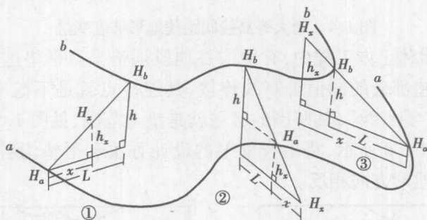
图 1.2 插入法求任意点高程图示
