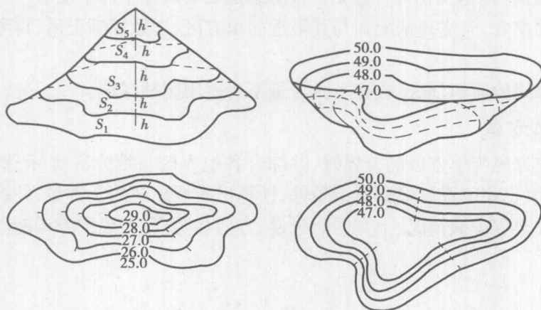
图 1.11 等高面法
