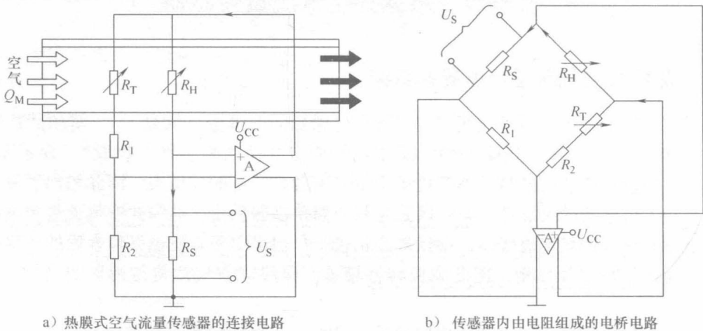
图 2-2 热膜式空气流量传感器电路
