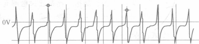
图 1-2 磁电式传感器产生的交流信号波形
