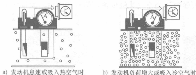
图 2-3 热膜式空气流量传感器的测量原理
