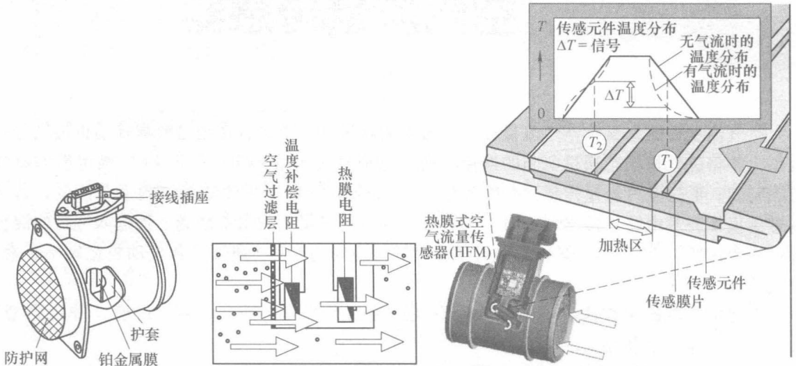
图 2-1 热膜式空气流量传感器的结构
