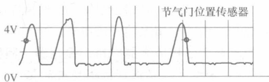
图 1-1 非恒压直流信号波形
