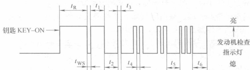
图 1-3 串行数据信号波形
