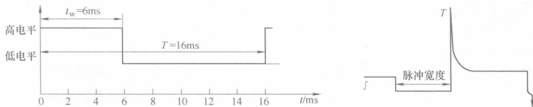
图 1-4 脉宽调制信号波形
