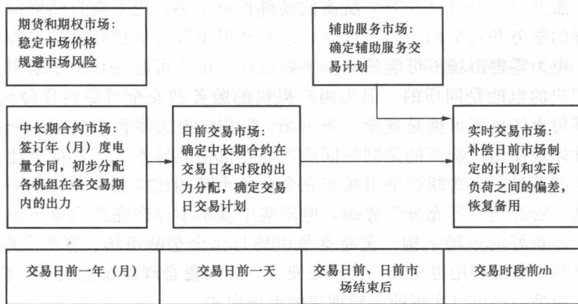
图 1-1 电力市场运作时间关系图
