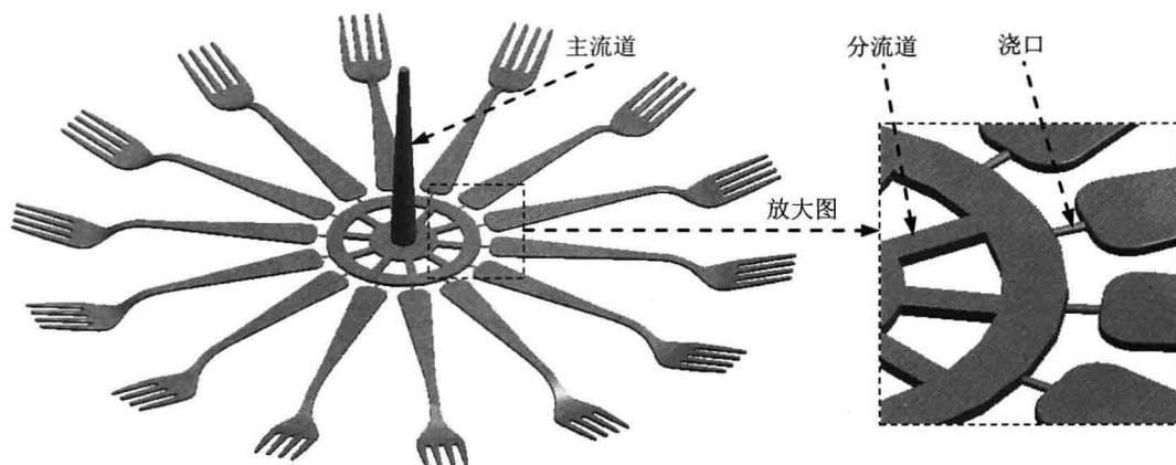
图 1.1.5 浇注系统
