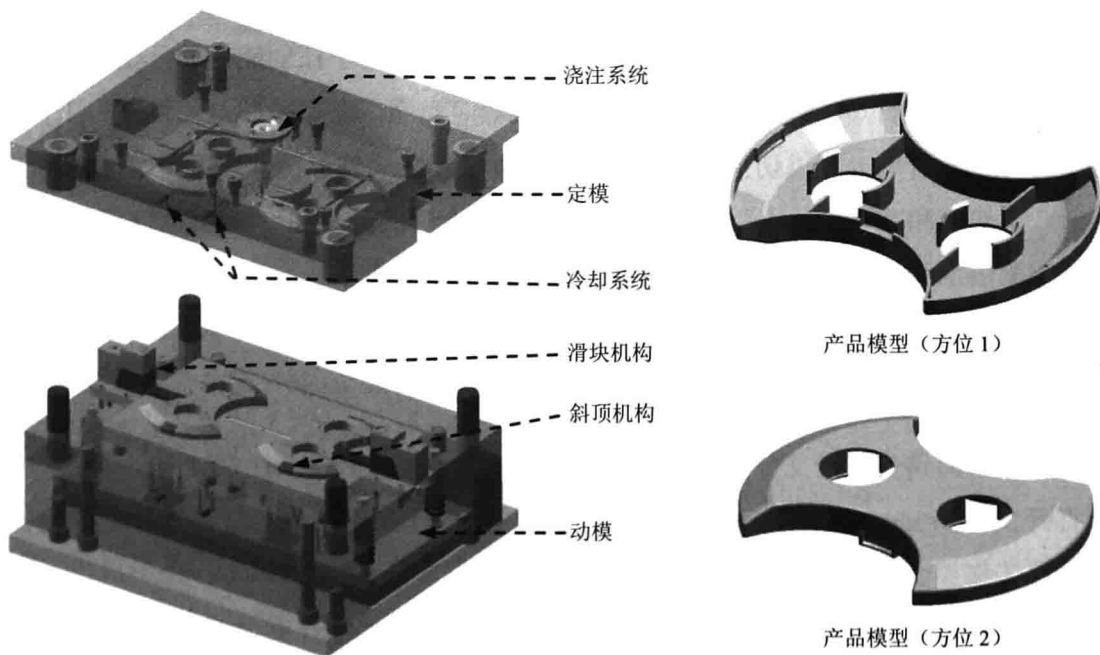
图 1.1.6 模架设计
