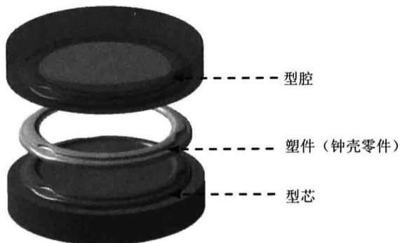
图 1.1.1 塑件成型元件
