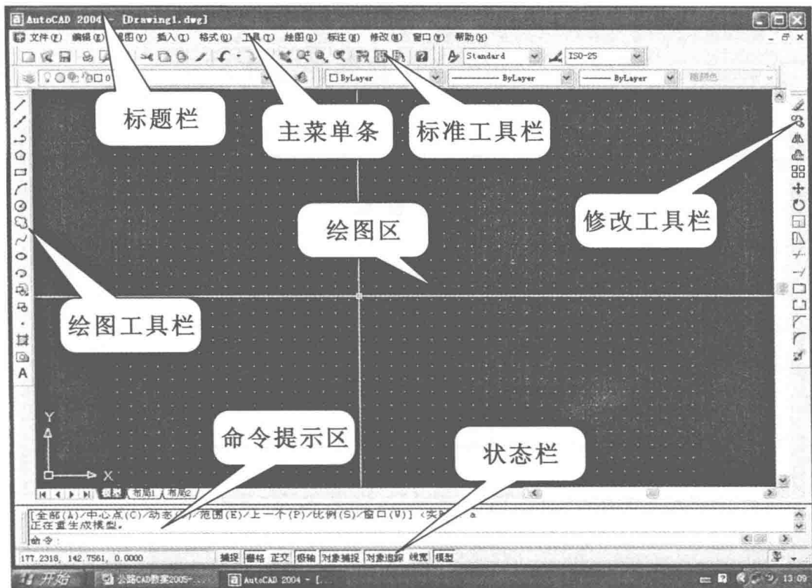
图 1-1-1 AutoCAD 软件的工作界面
