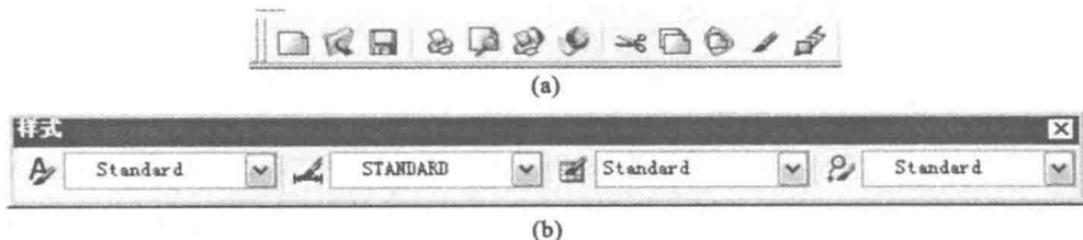
图 1-1-2 工具栏状态
