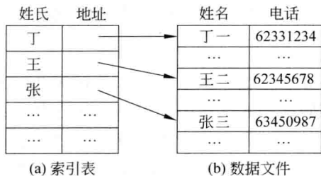
图 1.7 索引存储
