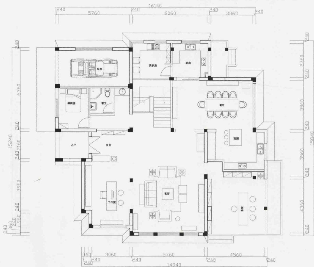
一层平面图
