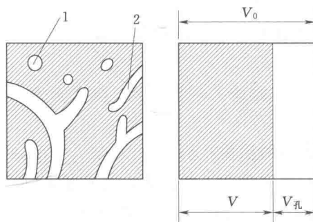
图 1.1 块状材料体积构成示意图
