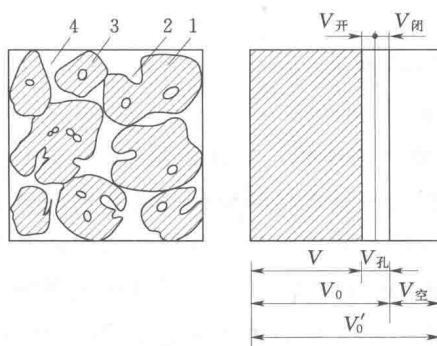
图 1.2 散粒材料体积构成示意图
