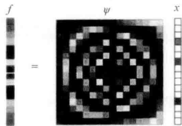
图 2-2 用基 \psi 进行稀疏表示(3 稀疏度)
