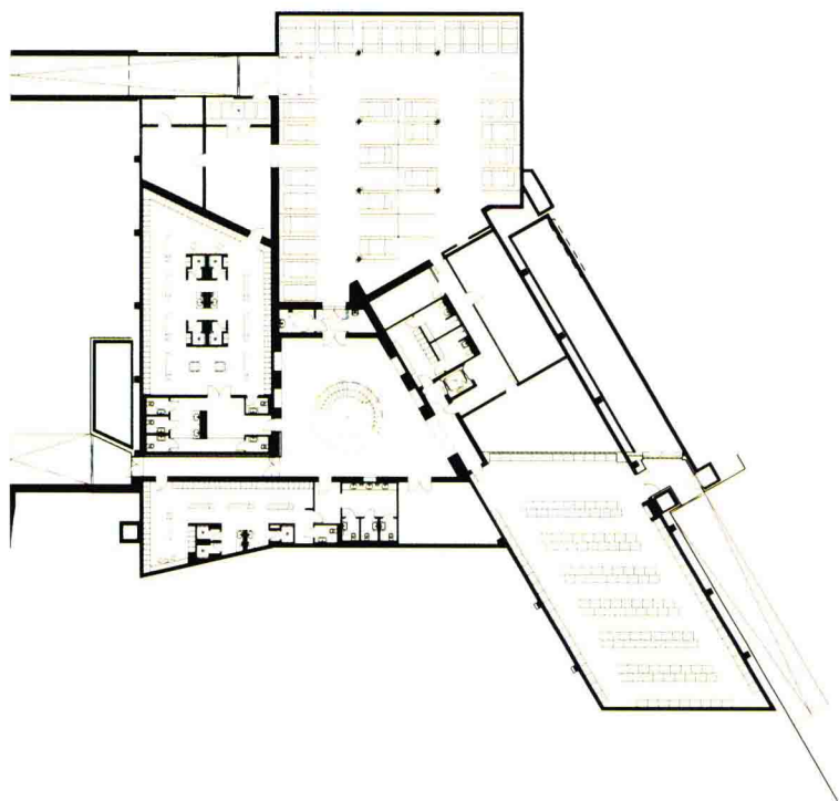
一层平面图
