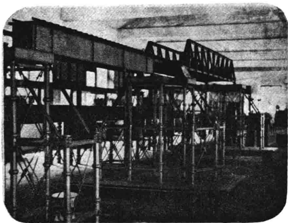
汉平路黄河铁桥模型（蒋汉澄摄于交通陈列馆）。
