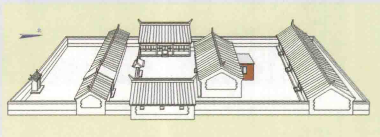
根据实地考察情况绘制的八道湾 11 号院落。不难看出模型与实际情况的差别。
