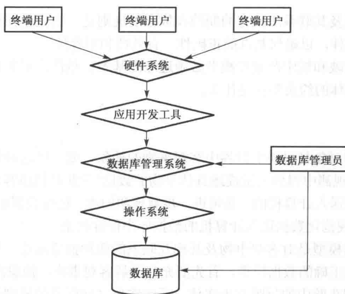
图 1.4 数据库系统组成示意图
