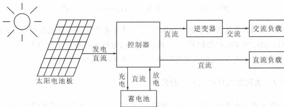
图 1-10 独立型太阳能光伏发电系统的工作原理
