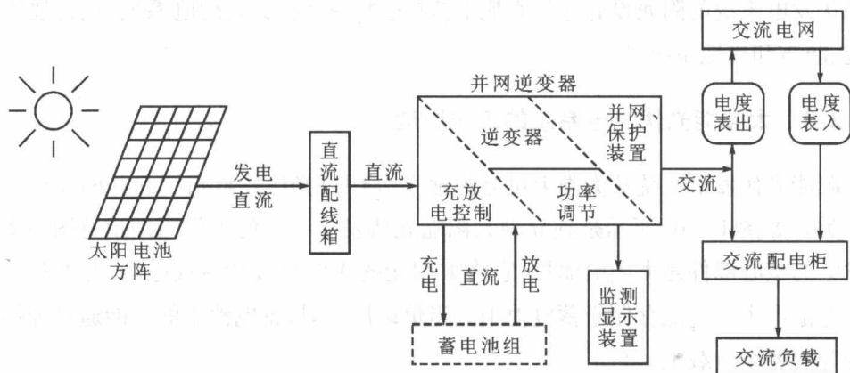
图 1-11 并网型太阳能光伏发电系统的工作原理
