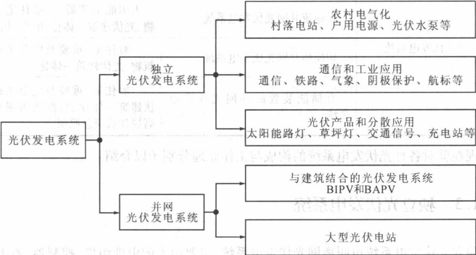
图 1-12 太阳能光伏发电系统的分类
