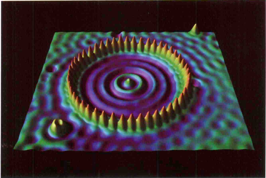
图3 由48个铁原子在铜表面围成直径为14.3纳米的“量子围栏”的STM图像。围栏中电子无法逃逸，在其中形成同心圆状的驻波，这是世界上首次观察到电子驻波的直观图形（见正文 § 4.2和 § 4.5）
