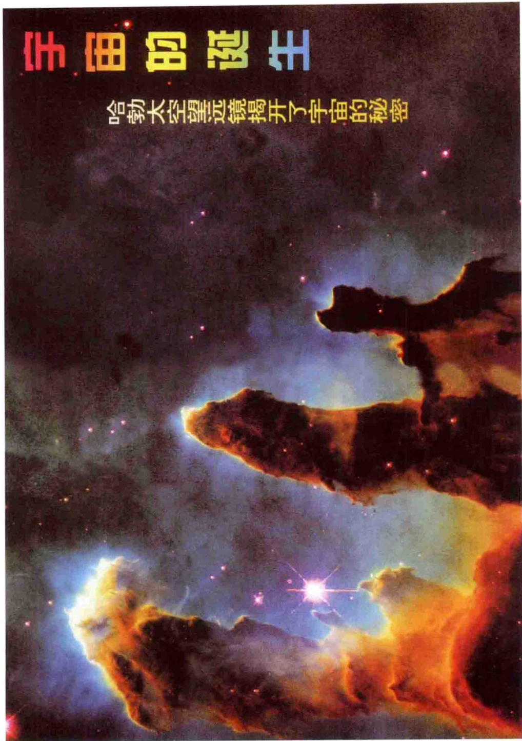
图7 哈勃太空望远镜所观察到的离地球七千光年的鹰状星云，它是新生星体的摇篮。这里到处是一缕一缕卷曲的星际氢气，每个气柱的厚度约等于太阳系的宽度（见正文 § 9.5）
