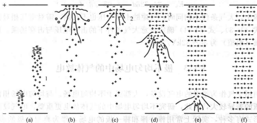
图 1-4 正流注的产生及发展
