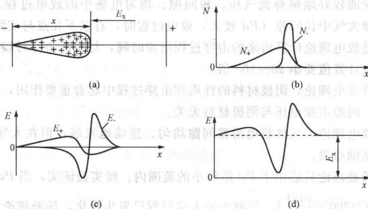
图 1-3 平行板电极间电子崩空间电荷对外电场的畸变作用
