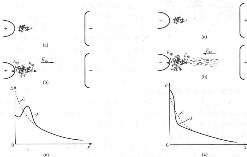
图1-5 正棒—负板间隙中非自持放电
