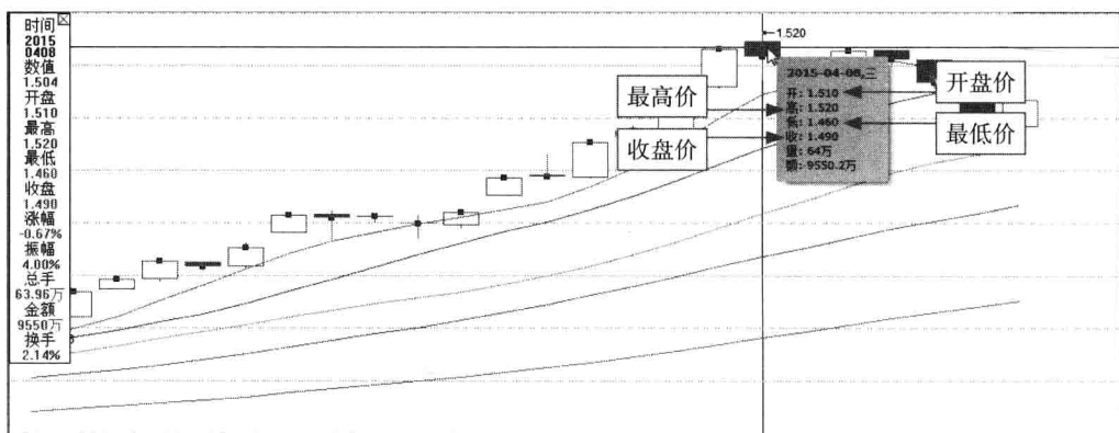
图 1-3 K 线图
