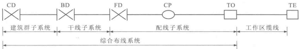
图 1.1 综合布线系统构成
