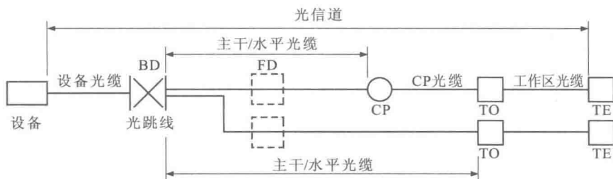
图 1.6 光纤信道构成(三)(光缆经过电信间 FD 直接连接至设备间 BD)
