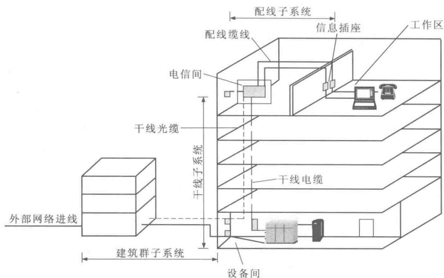
图 1.2 综合布线系统各组成部分示意图
