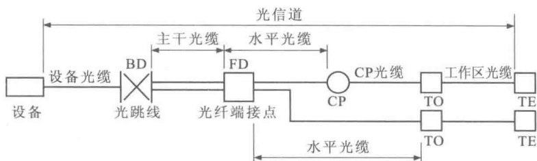
图 1.5 光纤信道构成(二)(光缆在电信间 FD 做端接)
