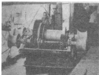
民生实业公司轮船“民元”轮上可负载 17 吨的起重设备在厂矿内迁中发挥了重要作用
