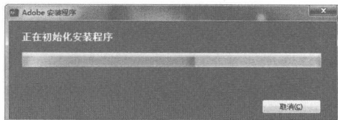
图1-2 初始化程序
