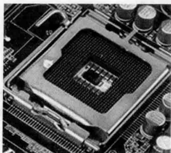
图 1-7 LGA 775 插座
