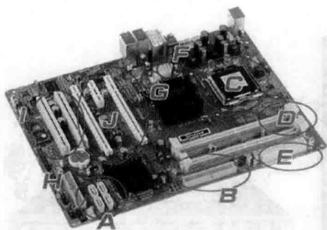
图 1-6 主板
