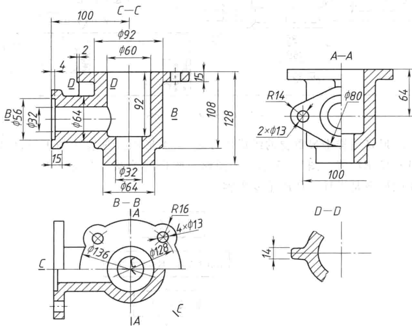
图 1-5 三通管视图
