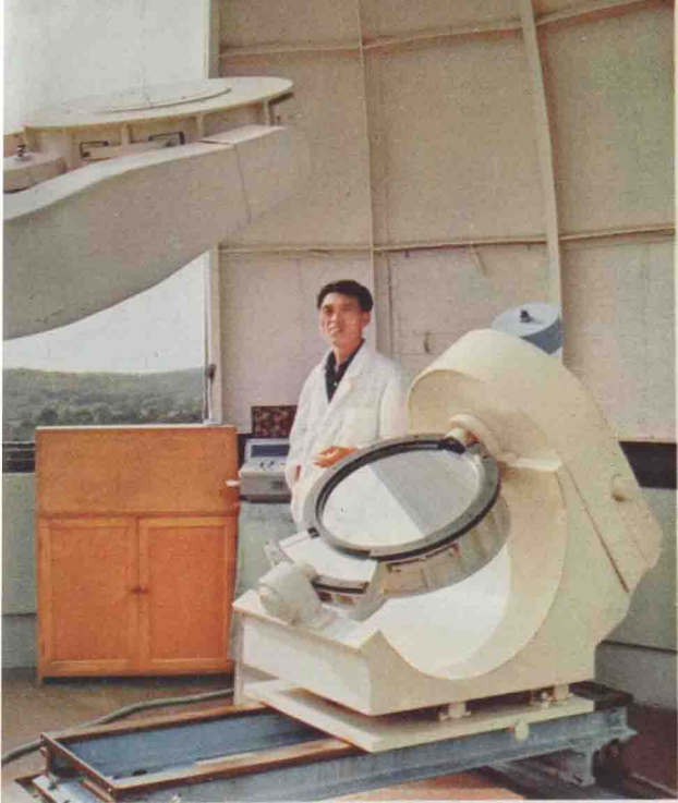
太阳塔的主要部件——定天镜
