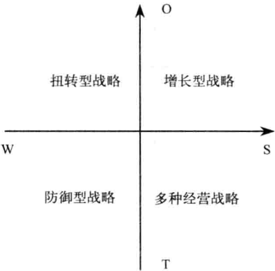
图 1-3 SWOT 分析法
