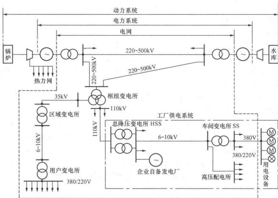
图 1-1 电力系统构成示意图
