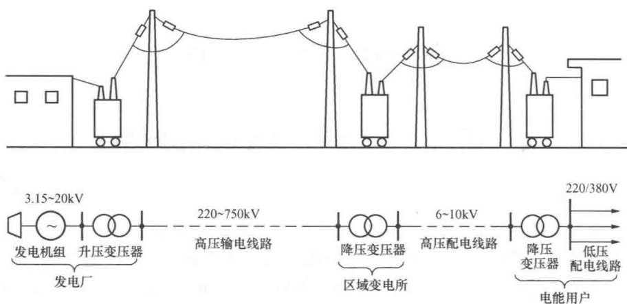
图 1-2 从发电厂到用户的发、输、配电过程示意图
