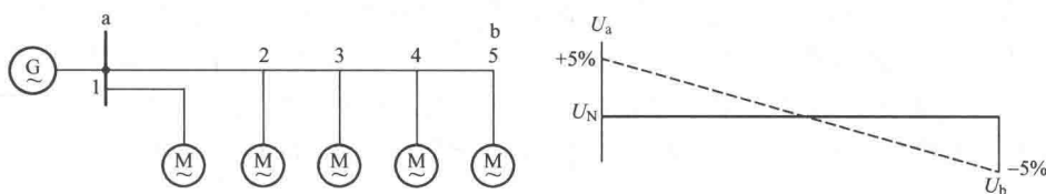
图 1-3 用电设备和发电机的额定电压说明
