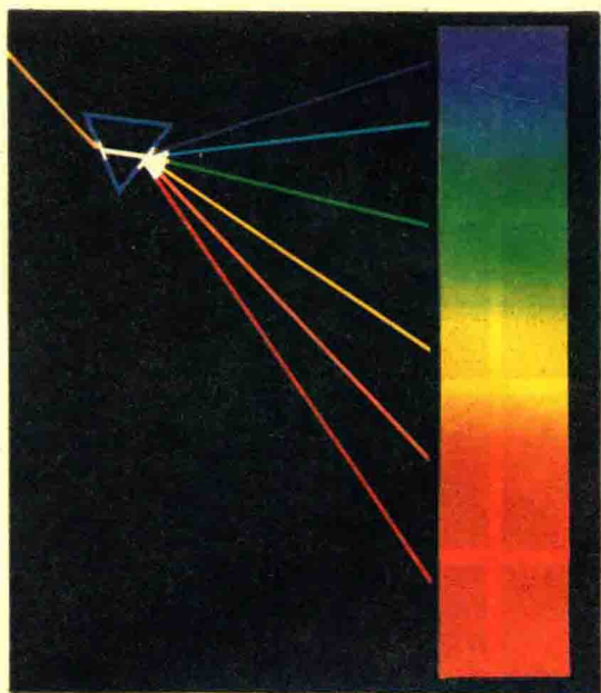
图 5 · 3 白光经三棱镜折射产生由红到紫的彩色光谱
