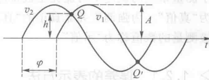
图 1-1-4 相位的测量方法
