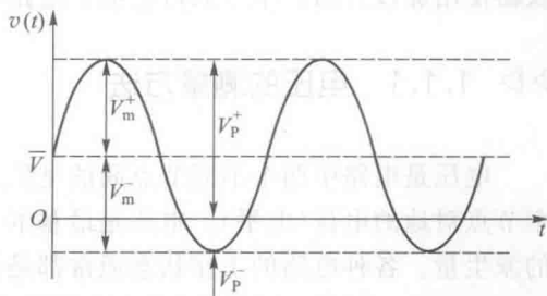
图 1-1-1 交流电压的量值
