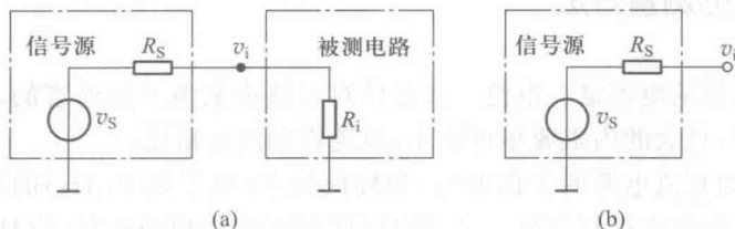
图 1-1-3 信号源的负载对输出电压的影响
