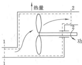
图 2-2 开口系统
