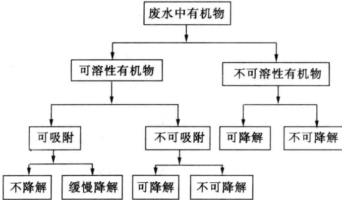
图 2-1 废水中的有机成分及其可处理性
