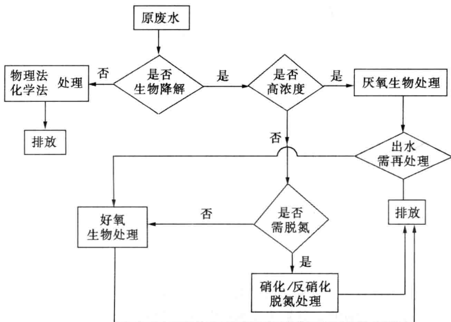
图 2-2 选择生物法处理的程序
