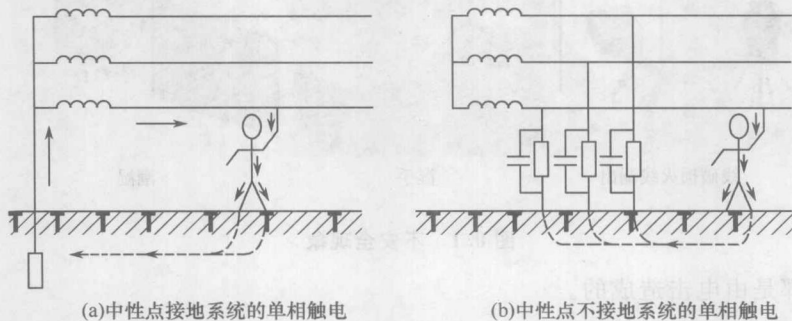
图 0.2 单相触电示意图
