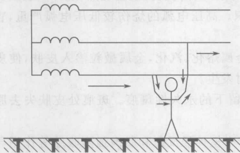
图 0.3 两相触电
