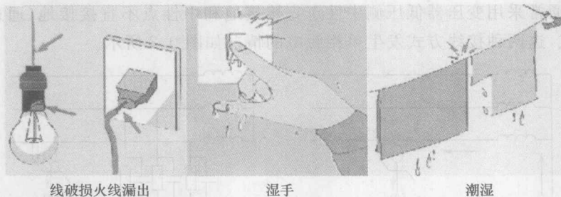
图 0.1 不安全现象
