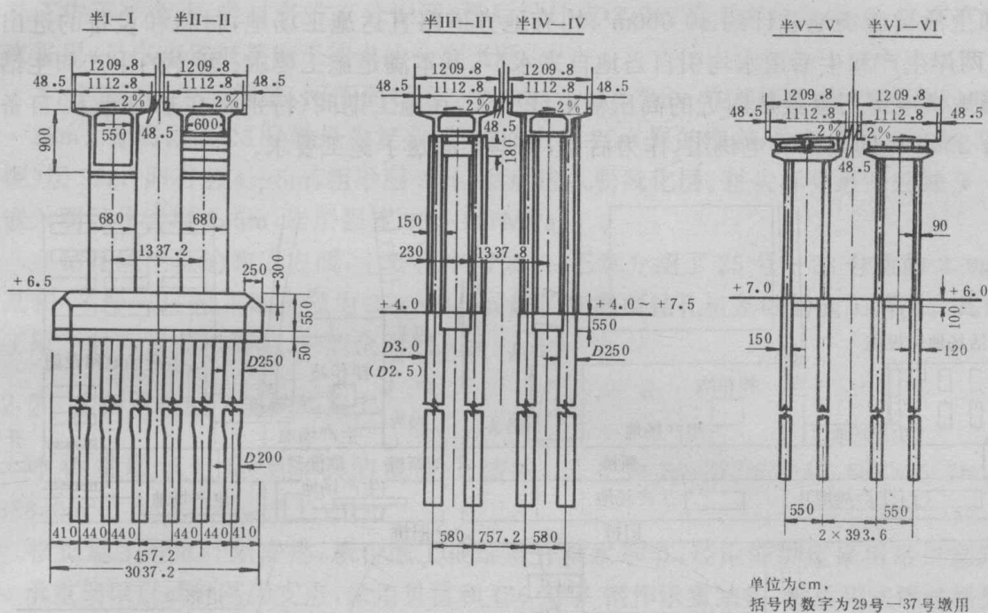
图1.3 九江大桥横断面布置
