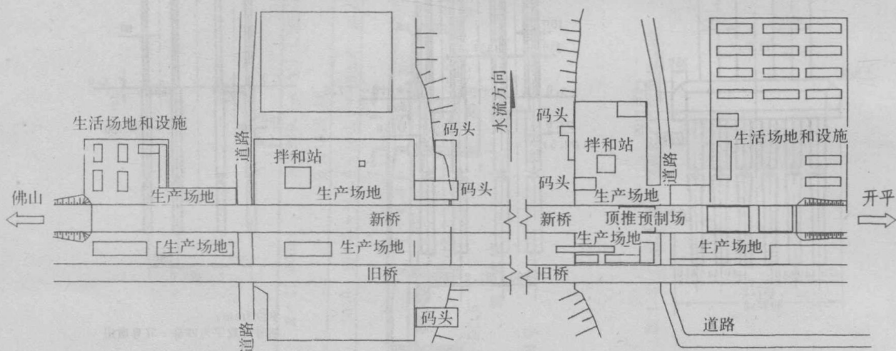
图 1.4 施工总平面布置图
