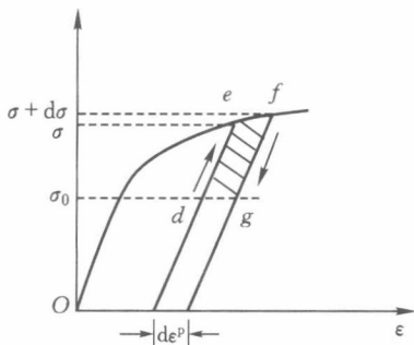
图 1.8 塑性功不可逆
