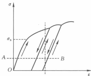
图 1.6 材料的强化特性
