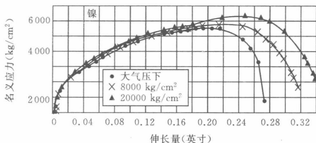
(a) 不同静水压力作用下镍的拉伸曲线
