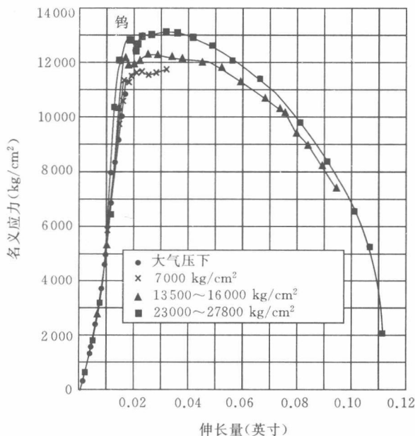
(b) 不同静水压力作用下钨的拉伸曲线
