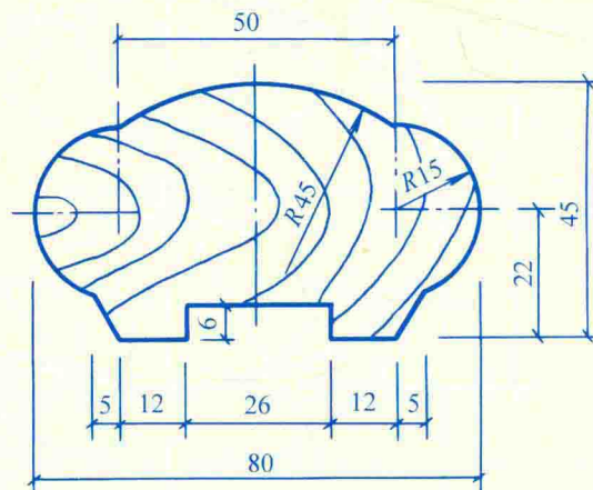
扶手 1:1
