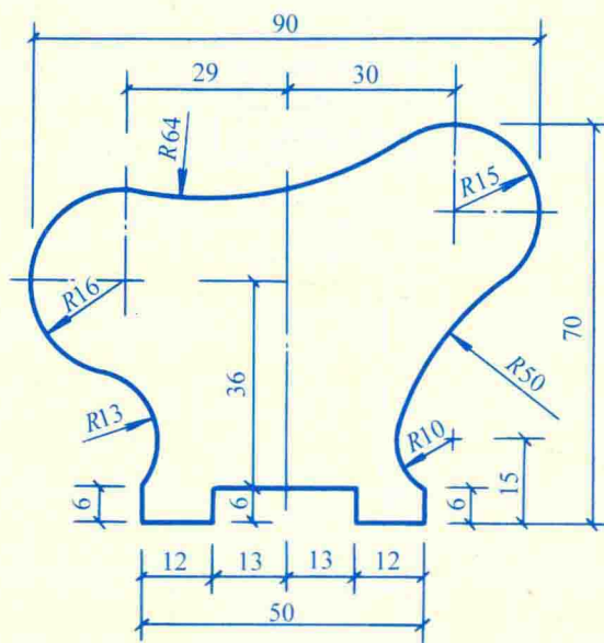
扶手轮廓 1:1
