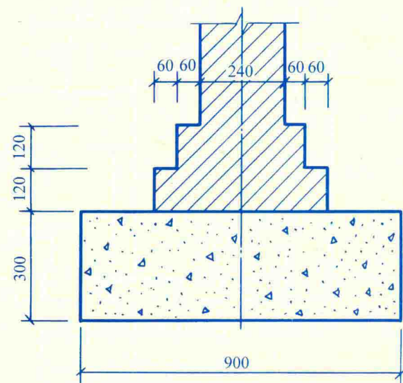
基础 1:10
