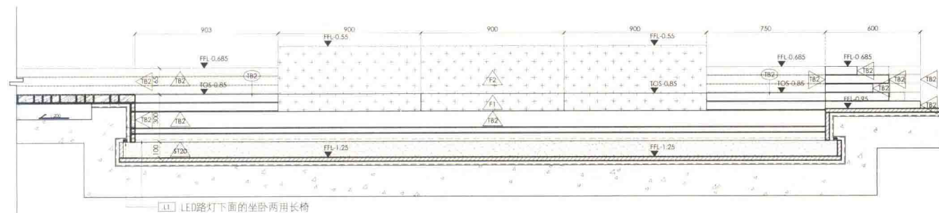
■ 立面图
