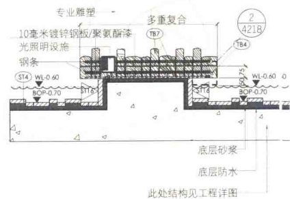
■ 剖面图
