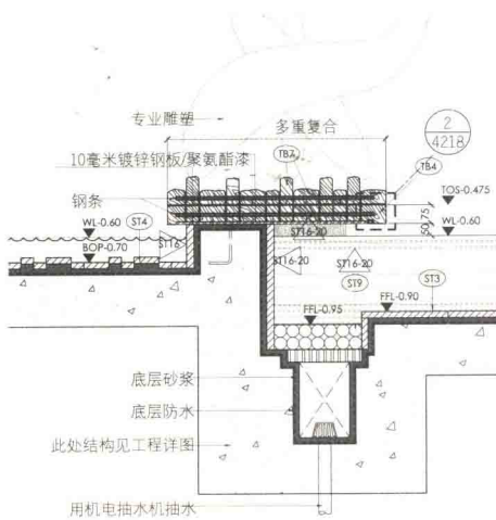
■ 剖面图
