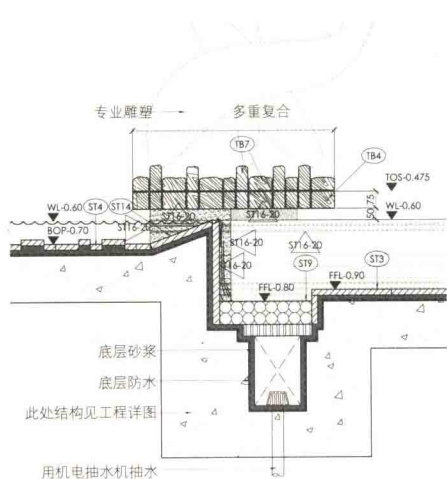
■ 剖面图
