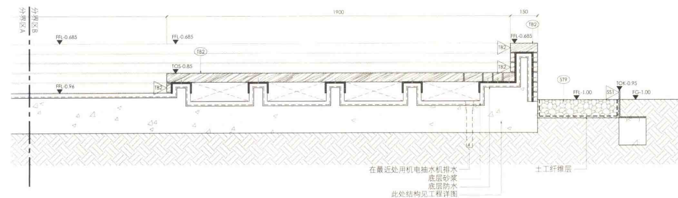
■ 剖面C
