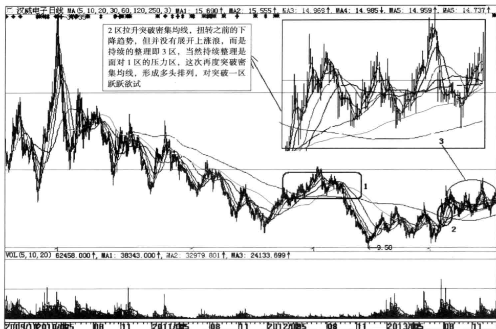
图 1-3 汉威电子 300007
