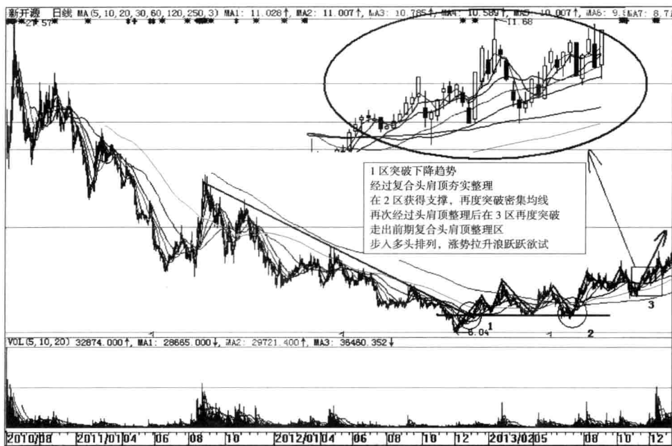
图 1-1 新开源 300109
