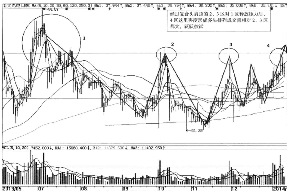
图 1-5 南大光电 300346
