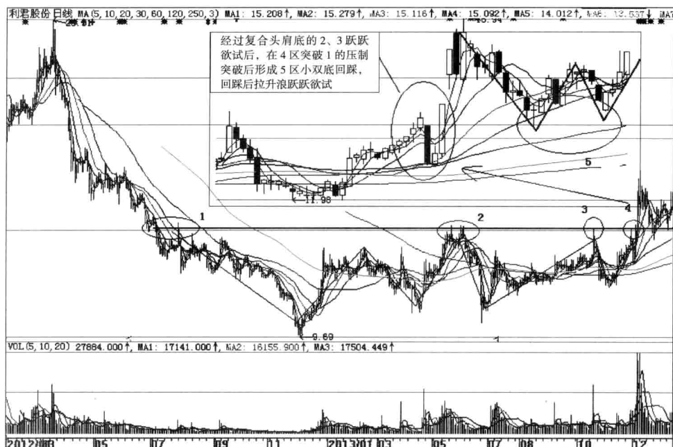
图 1-2 利君股份 002651
