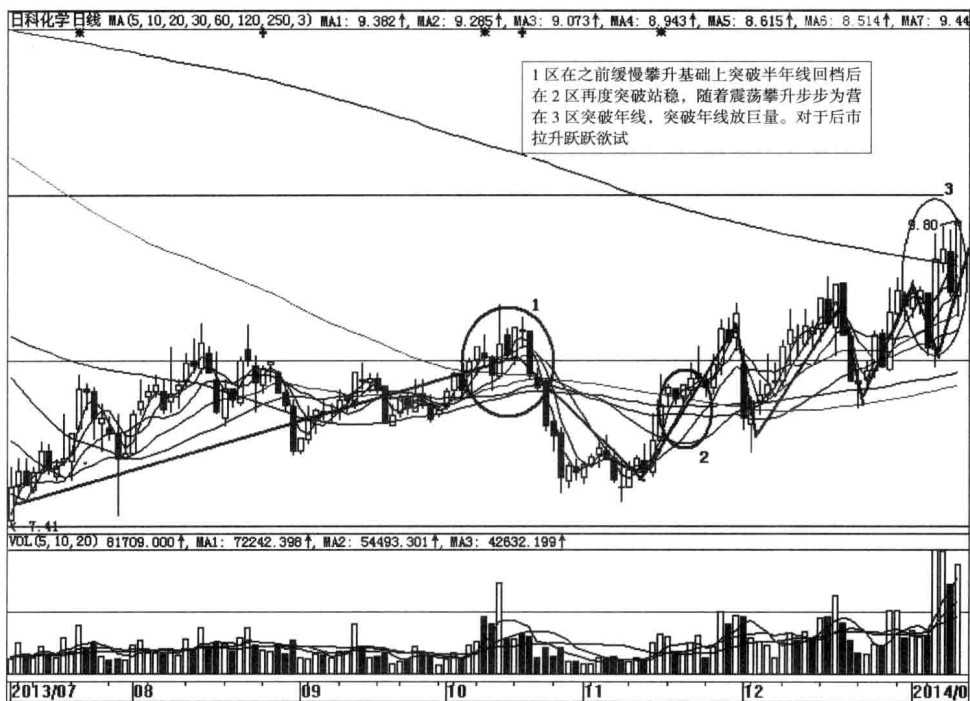
图 1-4 日科化学 300214
