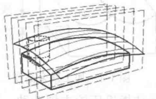
图 1-7 行切刀轨
