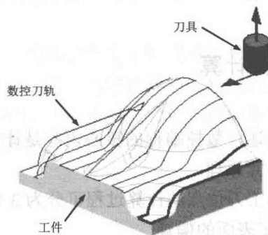
图 1-2 曲面加工
