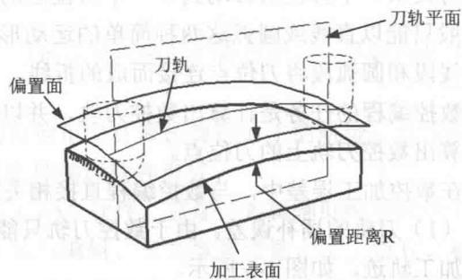
图 1-6 加工面偏置
