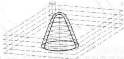
图 1-8 等高线刀轨
