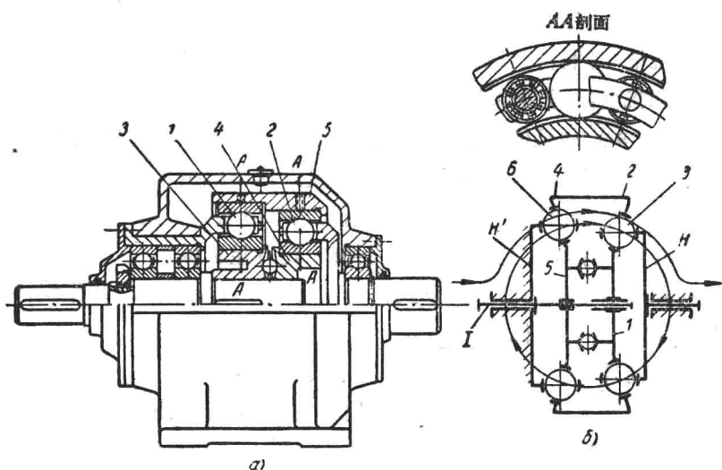
圖 5 內環具有自動壓緊裝置的滾珠式行星摩擦減速器的構造和傳動系統圖：
