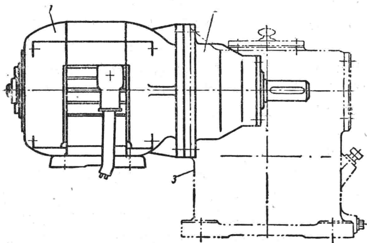
圖 1 滾珠式行星摩擦減速器的傳動裝置： 1—电动机；2—滾珠式減速器；3—蝸輪減速器。
