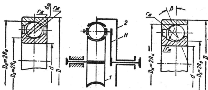
圖 2 徑向和徑向—止推軸承及其傳動系統圖:
